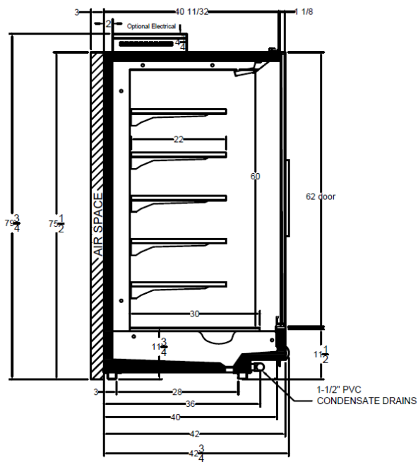
DX6UD CROSS VIEW
